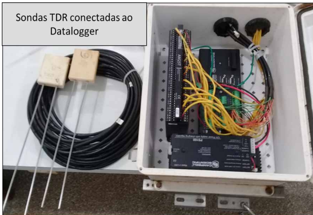
Figura 4 - Sensores TDR conectados ao Datalogger e bateria para armazenamento instantâneo da condutividade elétrica do solo.
