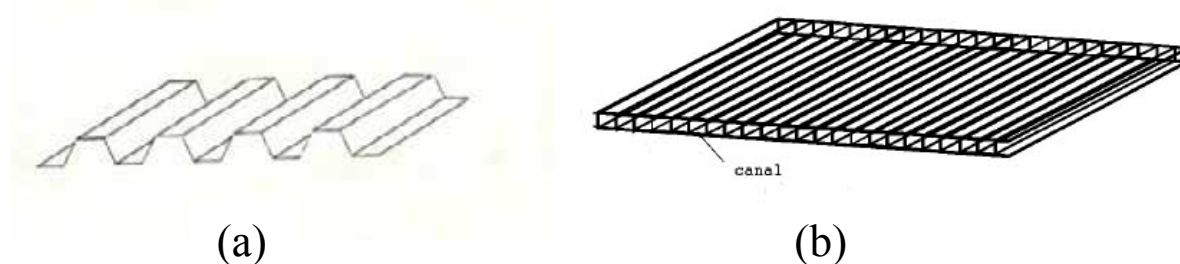
Figura 1 - Painel corrugado (a) e painel estruturado de parede dupla (b), utilizados em coberturas e em fechamentos laterais de abrigos para cultivo protegido.
