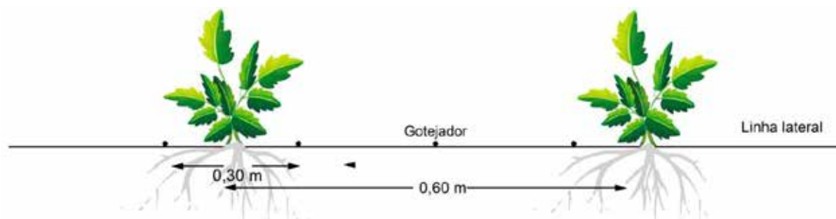
Figura 3 - Esquema da disposição dos gotejadores em linha lateral.
